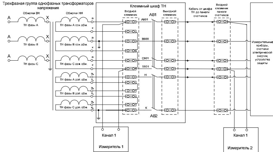
Рис. 2 Схема измерения потерь напряжения во вторичных цепях однофазных трансформаторов трехфазной группы. АВ1 - автоматический выключатель вторичных цепей основных измерительных обмоток; АВ2 - автоматический выключатель вторичных цепей дополнительных обмоток; А - X - выводы первичной обмотки ТН; а - х - выводы основных измерительных вторичных обмоток (звезда собрана на входном клеммнике); а д - х д - выводы дополнительных вторичных обмоток (разомкнутый треугольник собран на входном клеммнике); А01, В00, С01, 001; Н, К - маркировка основных и дополнительных вторичных цепей ТН;
